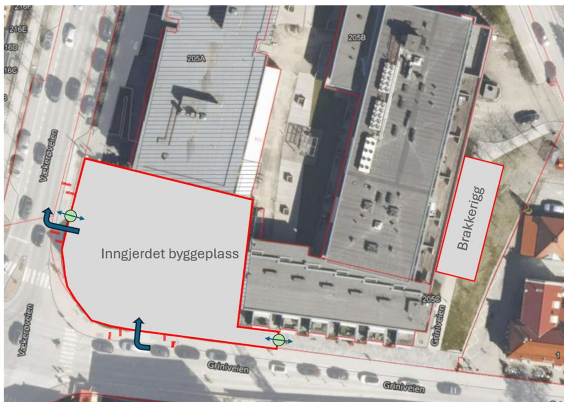
Figur 2 Riggplan Grunnarbeider
